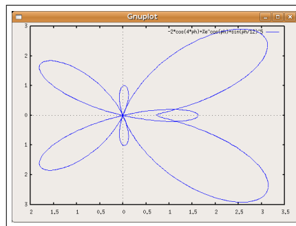
(d) r(\phi) = e^{\cos(\phi)} - 2\cos(4 * \phi) + \sin(\phi/12)^5
